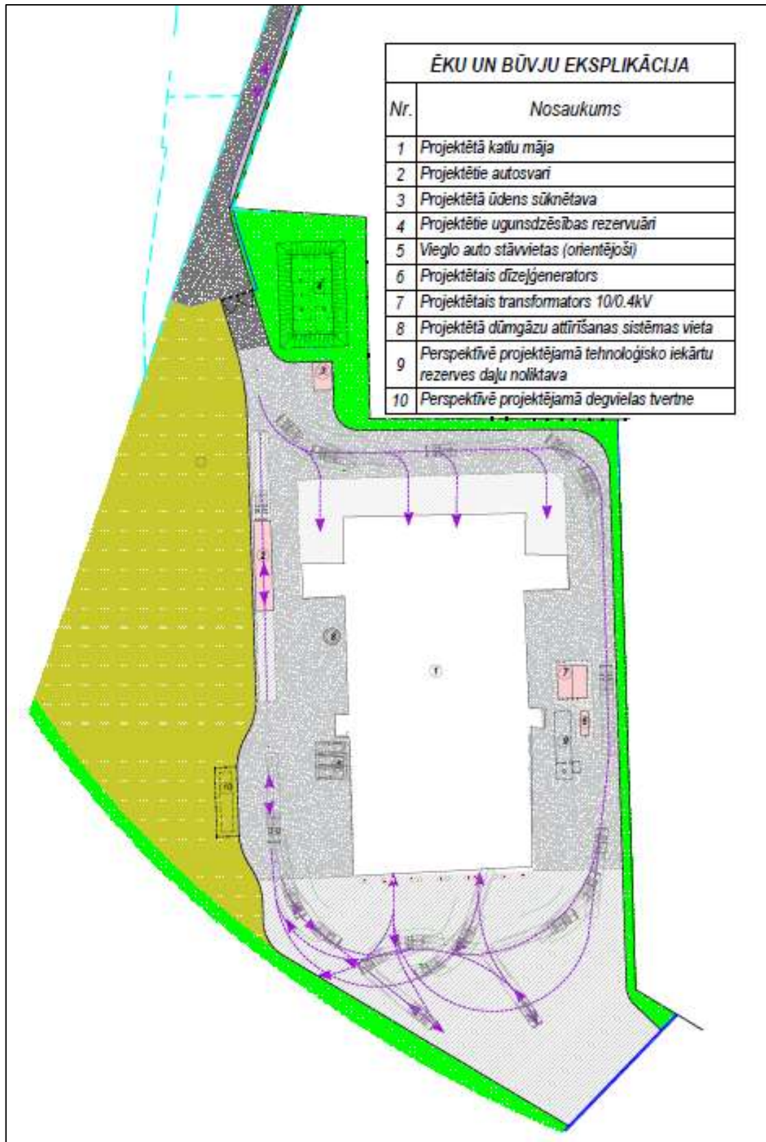
3.attēls. Paredzētās situācijas plāns ar objektu izvietojumu teritorijā
